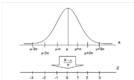
Figura A6-2 - Distribuição Normal típica normalizada
