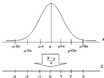
Figura A7-2 – Distribuição Normal típica normalizada
