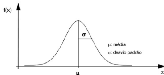
FIGURA A7-1 – DISTRIBUIÇÃO NORMAL TÍPICA
